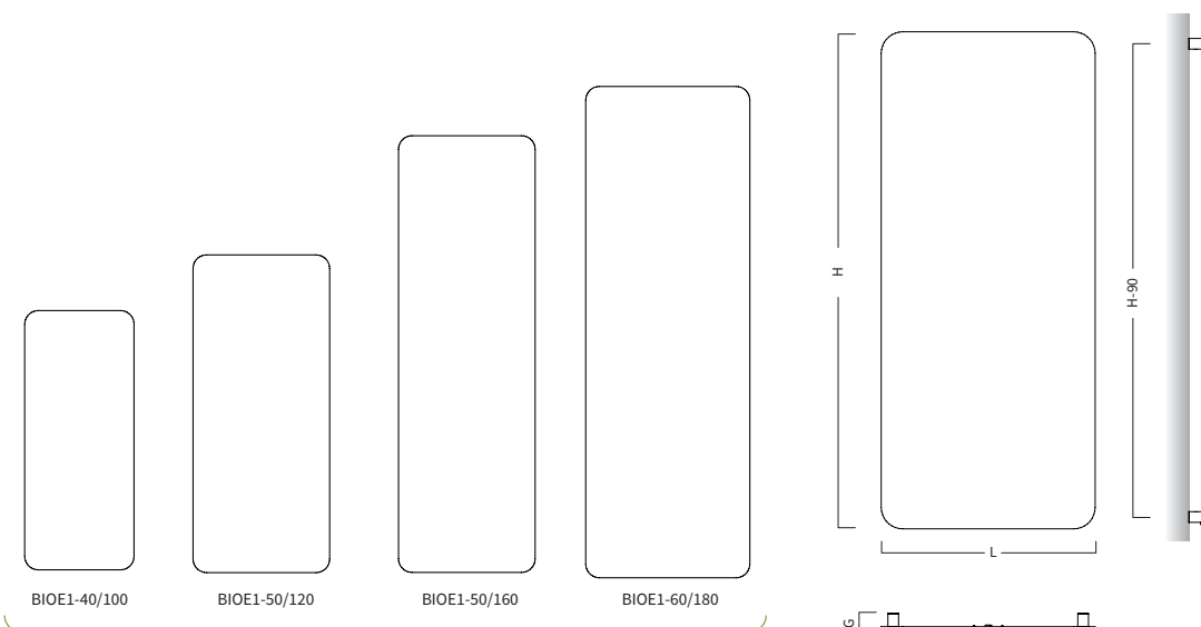
UKŁAD GRZEJNIKA ELEKTRYCZNEGO PRZY WYSOKOŚCI: electric radiator shape and design with the height:
