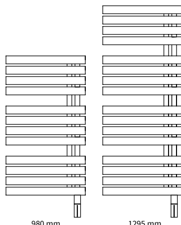
UKŁAD SUSZARKI PRZY WYSOKOŚCI: electric towel rail shape and design with the height:
